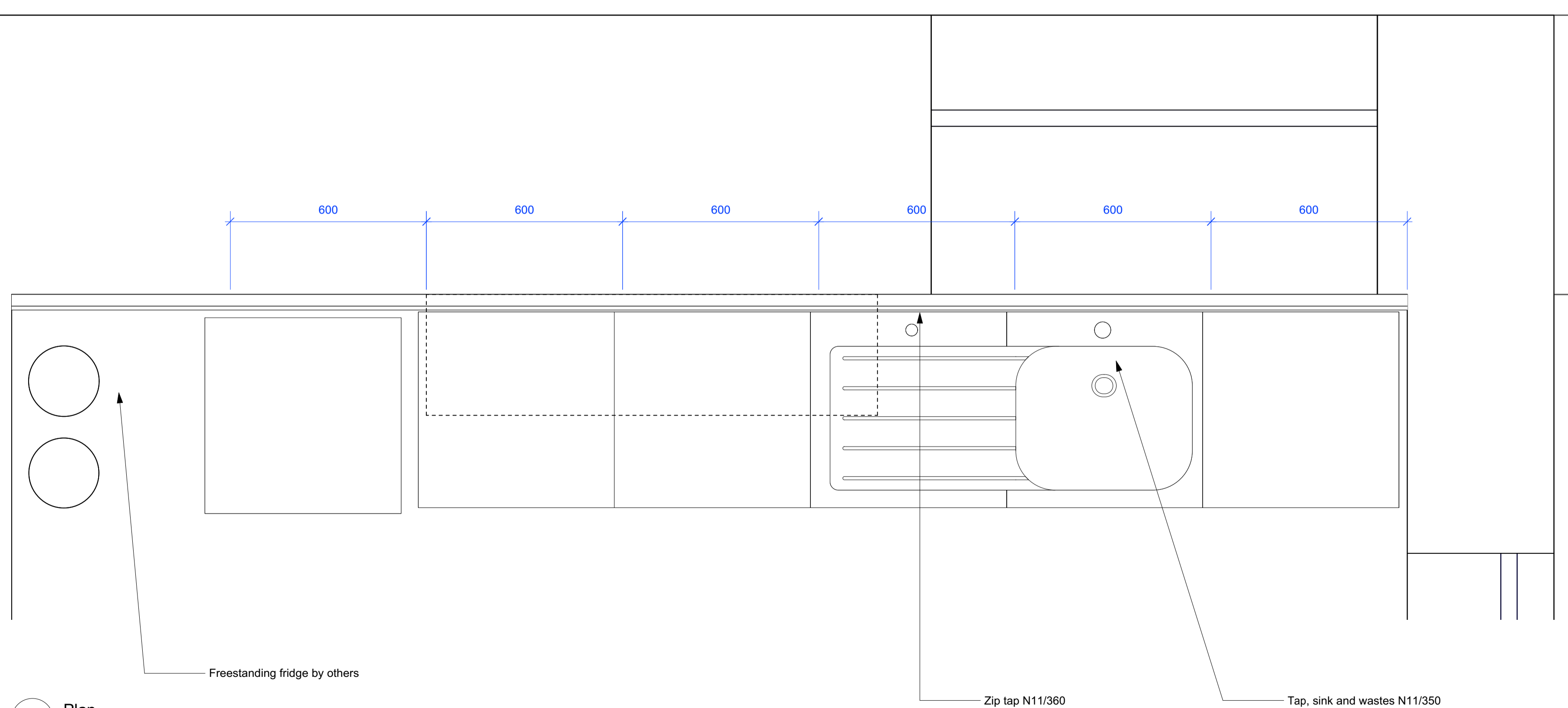
3 Plan Scale: 1:10
