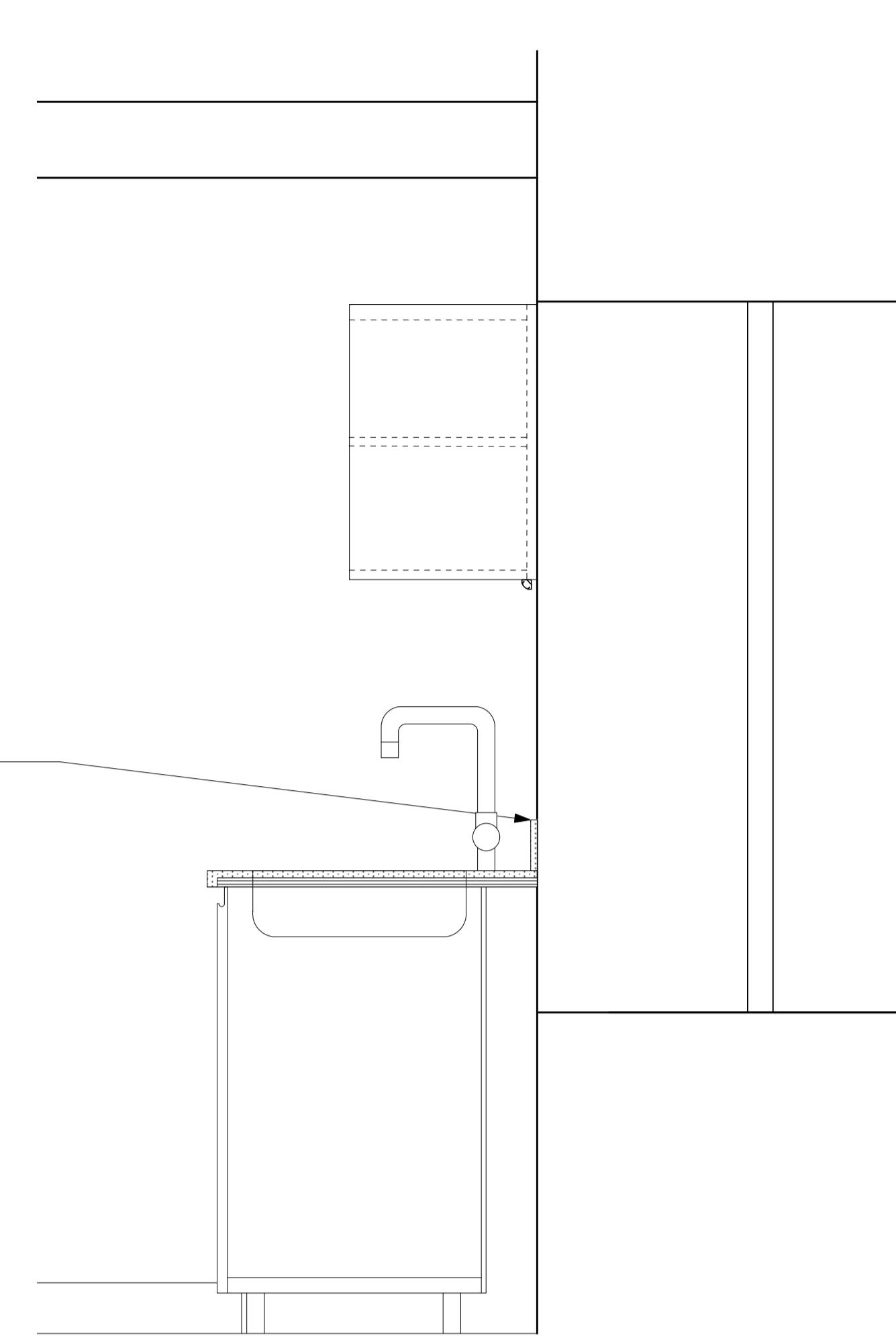
2 Section Scale: 1:10
