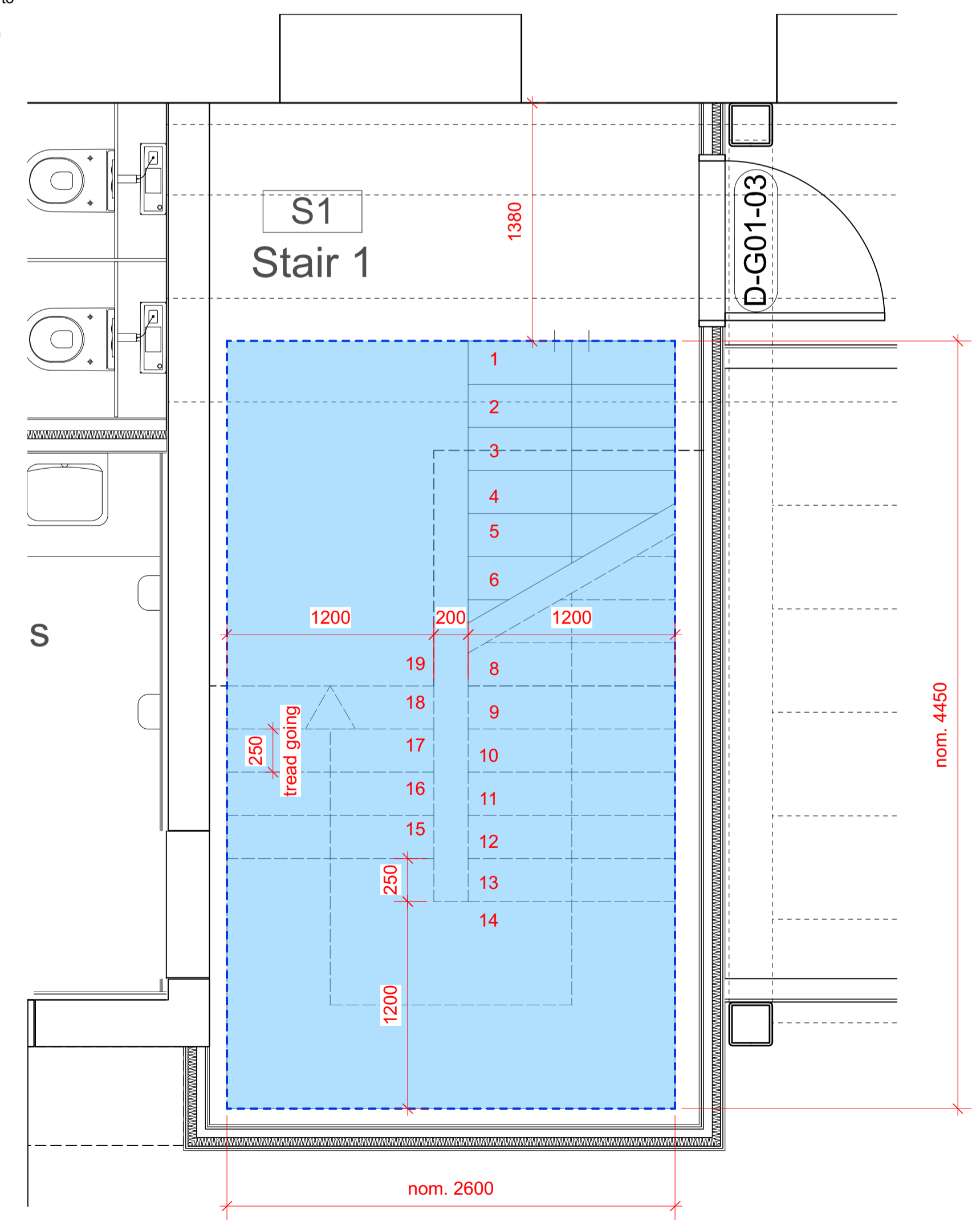
2 Stair 1 Plan Scale: 1:25
